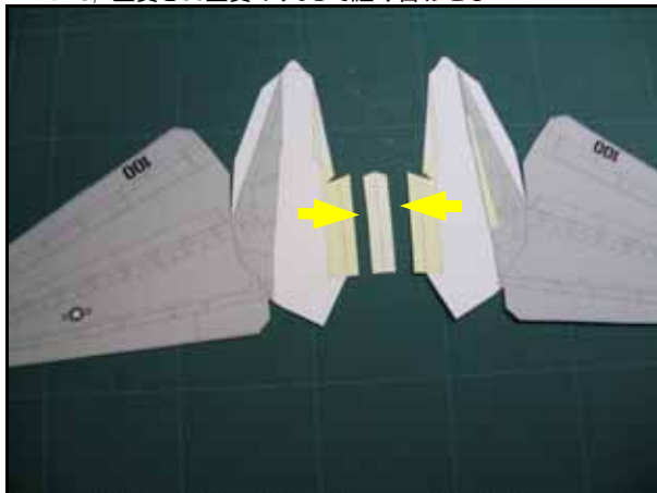
11. 主翼をのり付けする
