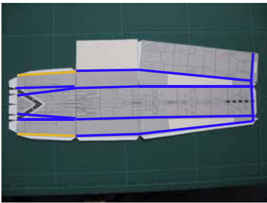
19 . G: 機体下部を組み立て、G2機体下部補強を内側にのりづけする
